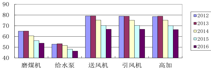
图 3-1 2012—2016 年五种辅助设备的可用系数 %
